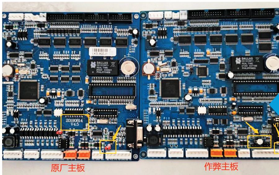
加油机原厂计控主板和非原厂主板对比图。(重庆市市场监管综合行政执法总队供图)
