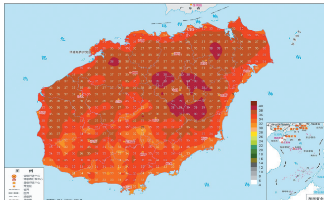
海南岛8月7日20时-8日20时最高温预报图。(来源:省气象局)
