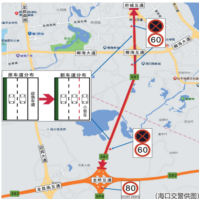
交通组织优化方案示意图
