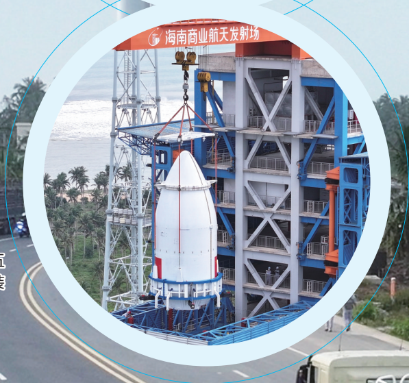
长八甲遥五火箭整流罩吊装作业现场。
